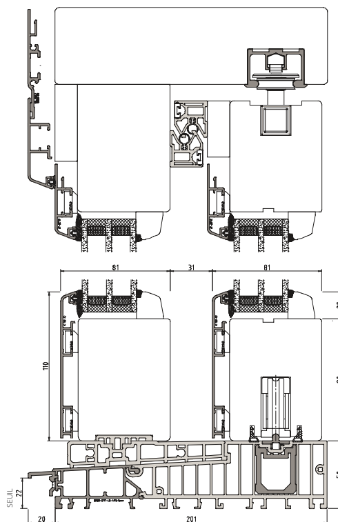
COUPE VERTICALE BAIE SOULEVANTE-COULISSANTE BOIS-ALU IDEALU IV 68
