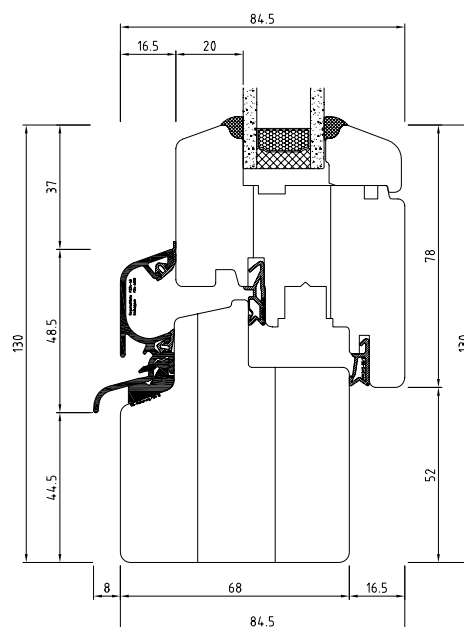
COUPE DE PROFIL DE FENÊTRE EN BOIS CLASSIQUE IV 68
