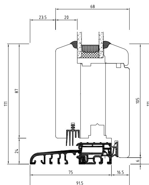
FENÊTRE EN BOIS CLASSIQUE IV 68 AVEC SEUIL PLAT
