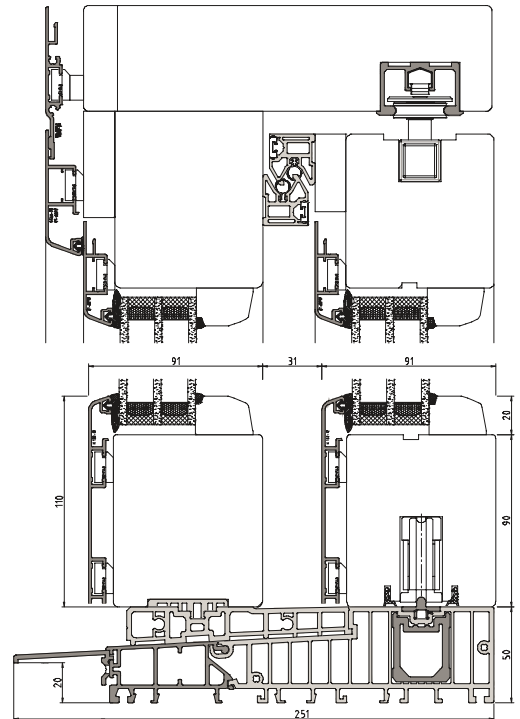
COUPE VERTICALE BAIE SOULEVANTE-COULISSANTE BOIS-ALU IDEALU IV 68 IDEALU VI 78
