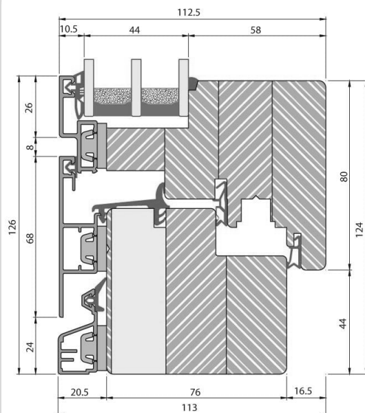
IDEAL ECO PLANO CHÂSSIS AVEC VANTAIL
