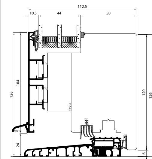
IDEAL ECO PLANO AVEC SEUIL PLAT
